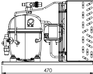
UNT6217Z
