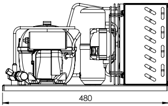
UEMT6144Z UEMT6170Z
